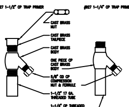
TYPICAL TRAP PRIMER DETAIL N.T.S.
